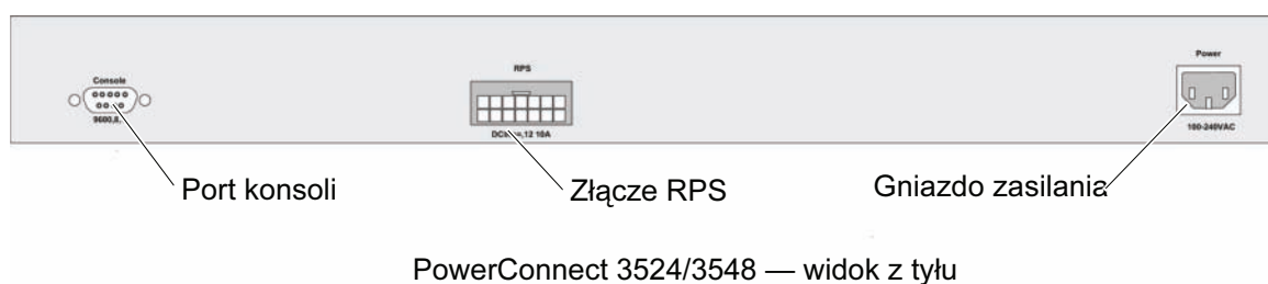
Rysunek 1-3. Złącze zasilania na panelu tylnym
